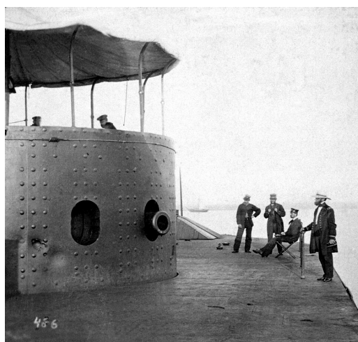
Башня «Монитора»
